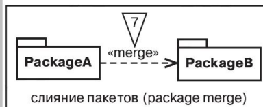
слияние пакетов (package merge)
