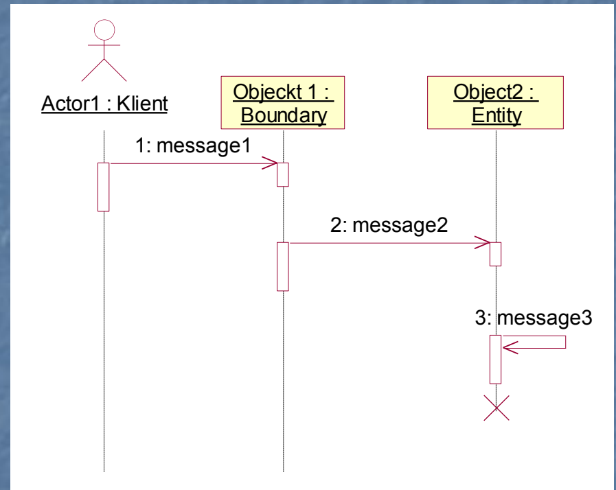
Sequence diagram – канонический вид
