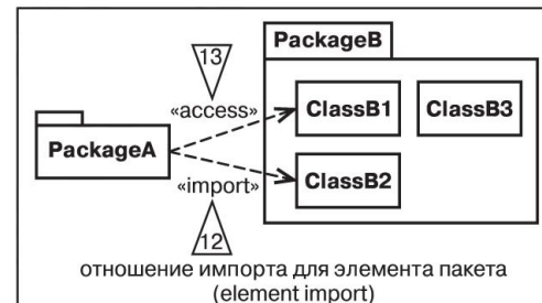
отношение импорта для пакета (package import)
